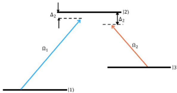
Рис. 1.1 Трехуровневая система активации лазерных импульсов
